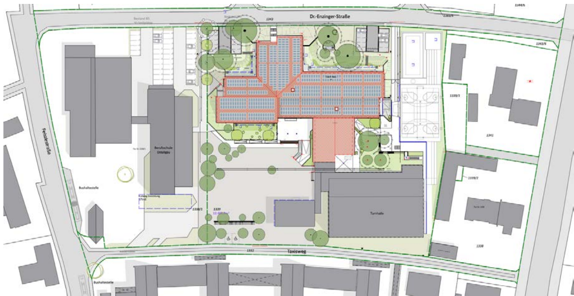
Abbildung 5: Lageplan, F64- Architekten, April 2025
