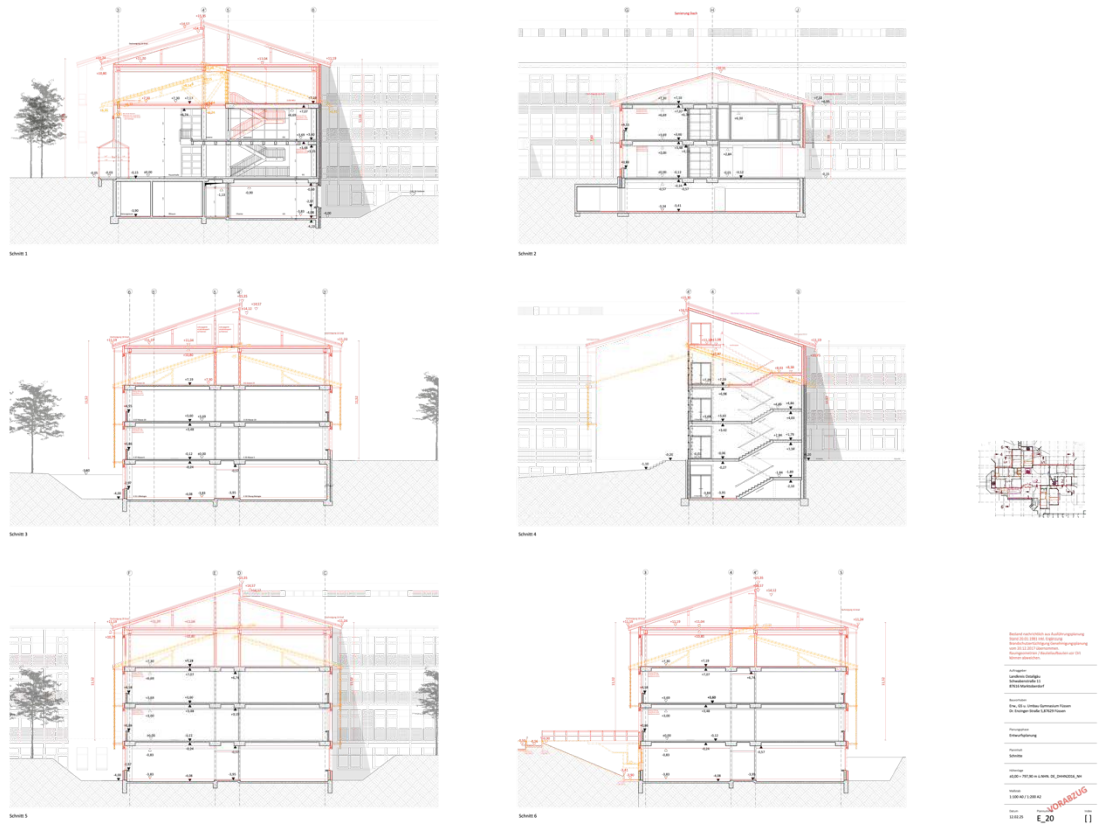
Abbildung 6: Schnitte, F64- Architekten, Februar 2025
