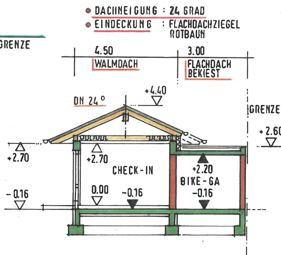
SCHNITT A-A
