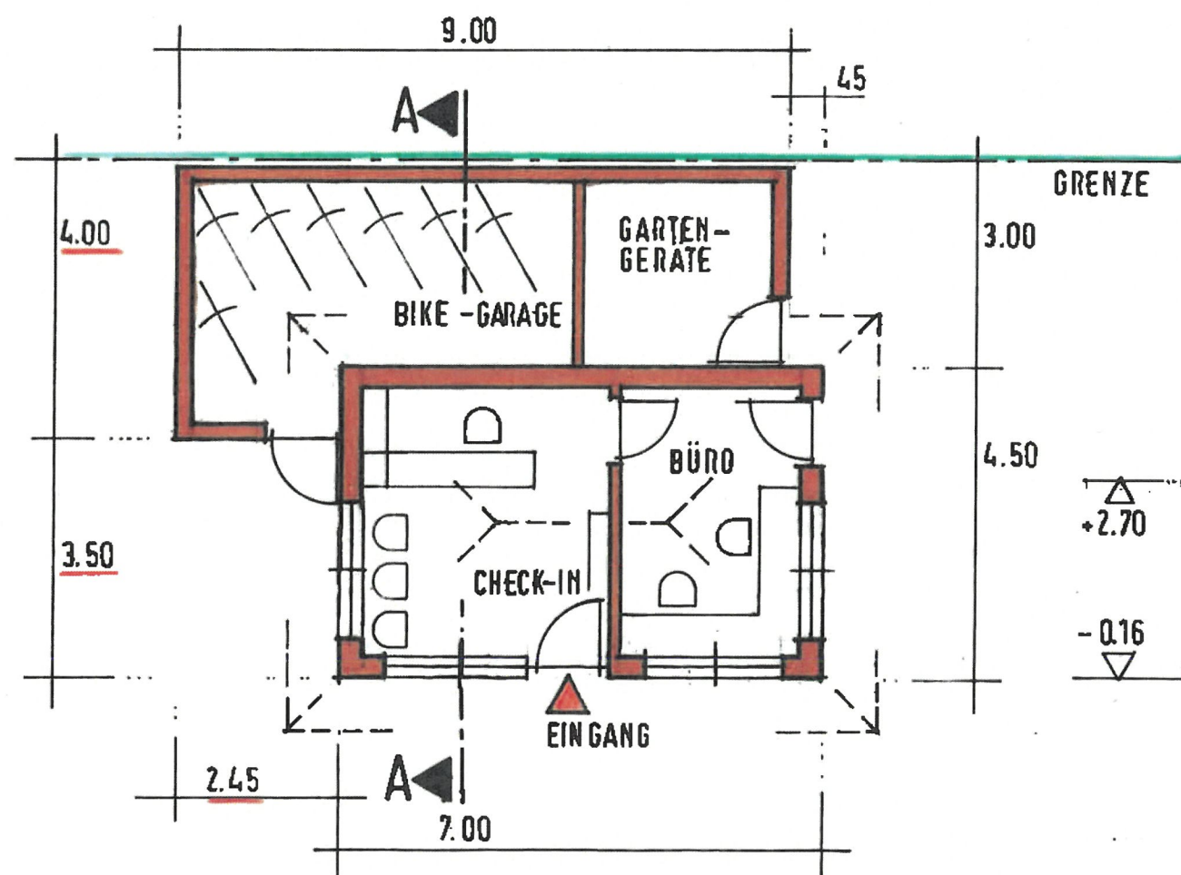
GRUNDRISS 1:100
